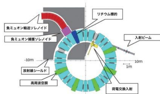
図 4 MERIT リングの基本構成
